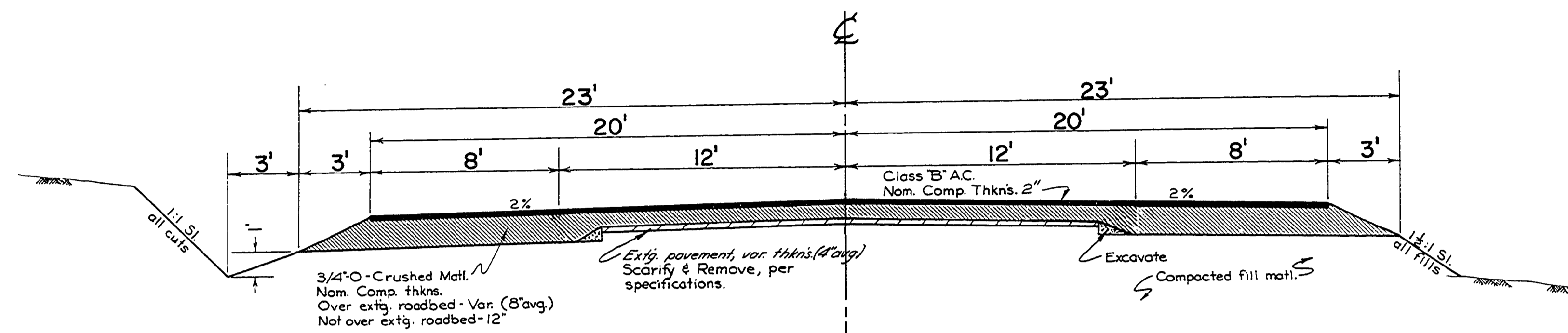
TYPICAL SECTION STA. 109+00 TO STA. 115+00 131+00 " " 137+00 196+00 " " 205+00
